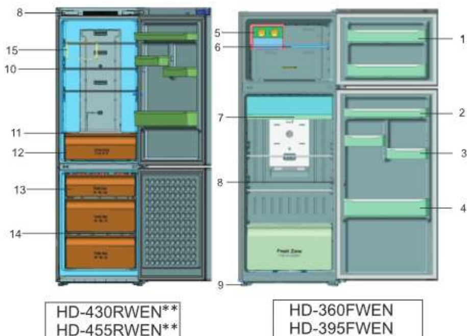
Расположение съемных и других частей холодильников
